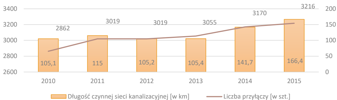
Wykres 12. Długość czynnej sieci kanalizacyjnej w latach 2010-2015 na terenie gminy [w km]
